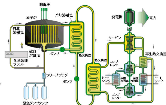
溶融塩炉 (MSR)
