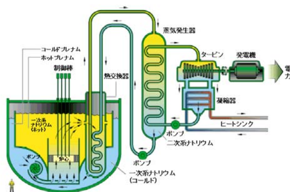
ナトリウム冷却高速炉 (SFR)
